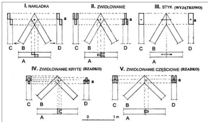
Rys. 60. Poprawne odwzorowanie więźby wymaga znajomości historycznych złączy. W kalenicy widoczne są tzw. sztorce i uciosy „a” rysujemy grubszą linią i nie zakreskowujemy. Należy pamiętać, że w kalenicy może się zmieniać kierunek połączeń. Oznaczenia: A – rzut więźby z góry, B – przekroje poprzeczne więźby, C i D – przekroje podłużne więźby (rys. J. Tajchman)
