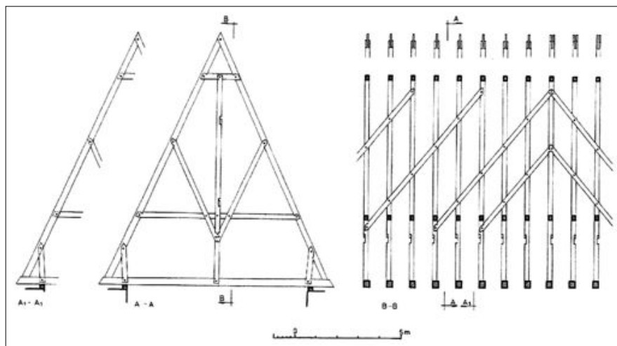
Rys. 59. Przekroje wykonujemy (pokazujemy) od strony odwiązywania, czyli bicia kołków, rysując złącza odpowiadające rzeczywistości. W przypadku konieczności „krojenia” z odwrotnej strony nakładki rysujemy linią przerywaną lub wykonujemy dodatkowy przekrój z widocznymi złączami (więźba jednostorczykowa nad nawą główną kościoła św. Jakuba z Torunia, ok. 1320 r.) (rys. ze zbiorów Zakładu Konserwatorstwa IżIK UMK w Toruniu wg J. Tajchmana)
